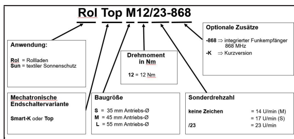
Fig. 13 RevoLine Bezeichnungserklärung
