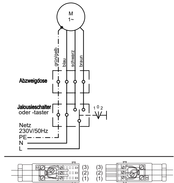
Fig. 5 Schaltbild RolTop 230 V / 50 Hz und Kabelbelegung bei Verwendung mit Hirschmann-Steckverbindung STAK-3 / STAS-3
